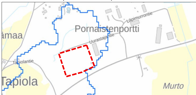
Kuva 3.9 Valuma-alue sinisellä
